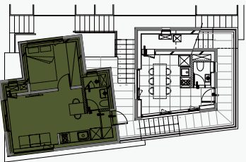
지상3층 평면도
