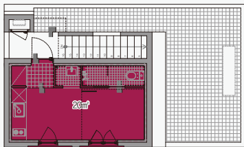
지상4층 평면도
